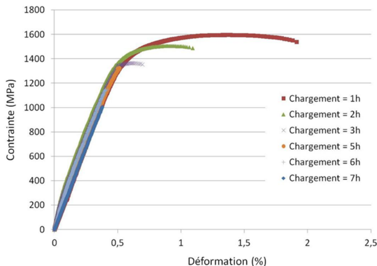
Figure 3 : Mise en évidence de la fragilisation par l'hydrogène par un essai de traction sur un acier durci et chargé en hydrogène entre 1h et 7h.
