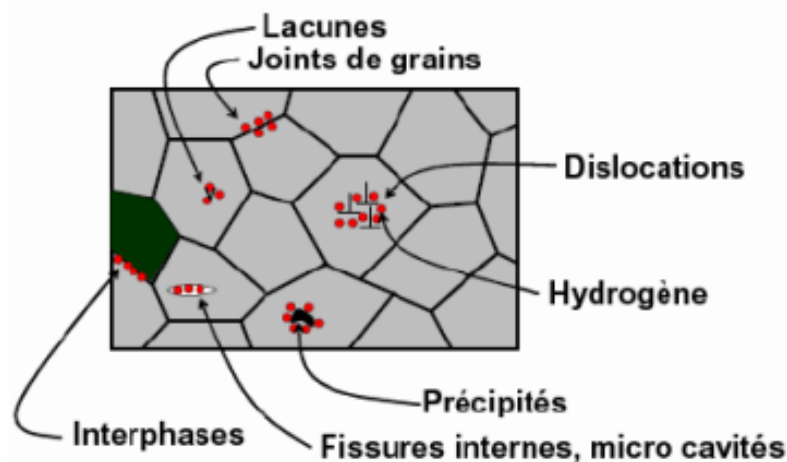
Figure 2 : Présentation schématique de différents types de défauts (ou sites de piégeage).
